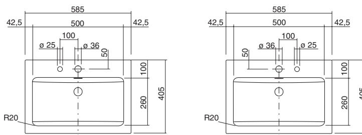
HB.S450H – mit Lotionspenderbohrung
