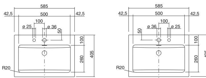
HB.R585H – mit Lotionspenderbohrung
