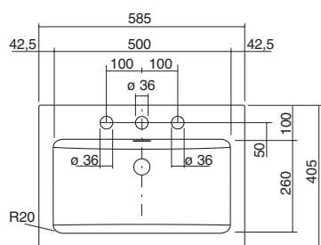
HB.R585H – mit 3 Hahnlöchern
