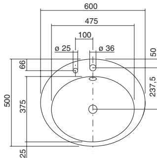
EB.0500H – mit Lotionspenderbohrung
