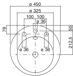
EB.0600H – mit 3 Hahnlöchern
