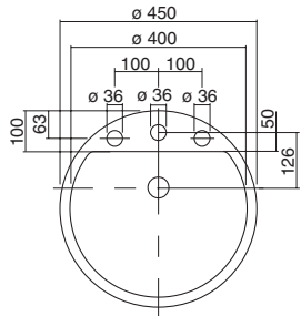
EB.K450H – mit 3 Hahnlöchern
