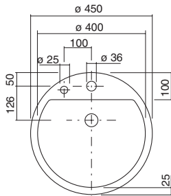
EB.K450H – mit Lotionspenderbohrung
