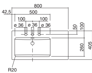
WT.PR800H3.R – mit 3 Hahnlöchern
