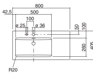
WT.PR800H.R – mit Lotionspenderbohrung
