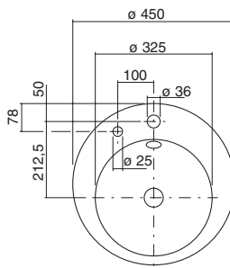
EB.0600H – mit Lotionspenderbohrung
