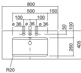
WT.PR800H3.L – mit 3 Hahnlöchern
