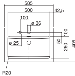
WT.PR800H – mit Lotionspenderbohrung
