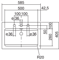
WT.PR800H3 – mit 3 Hahnlöchern
