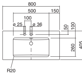
WT.PR800H.L – mit Lotionspenderbohrung
