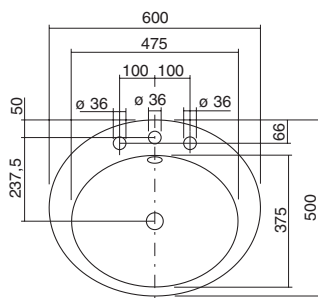
EB.0500H – mit 3 Hahnlöchern
